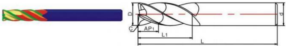
4-зубые концевые фрезы из карбида вольфрама для алюминия. Технические характеристики
